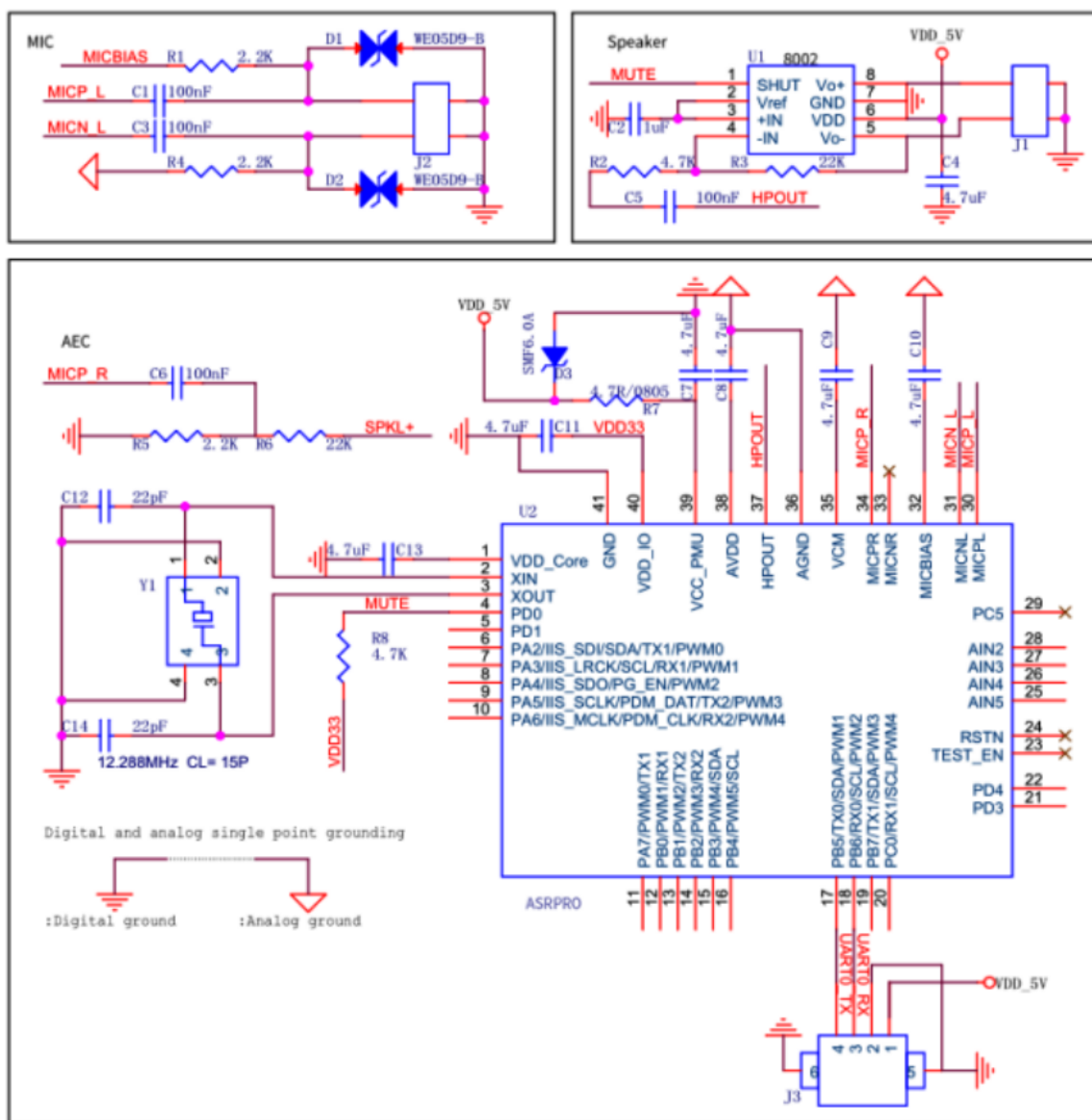
图 H-1 ASRPRO 应用参考电路图
